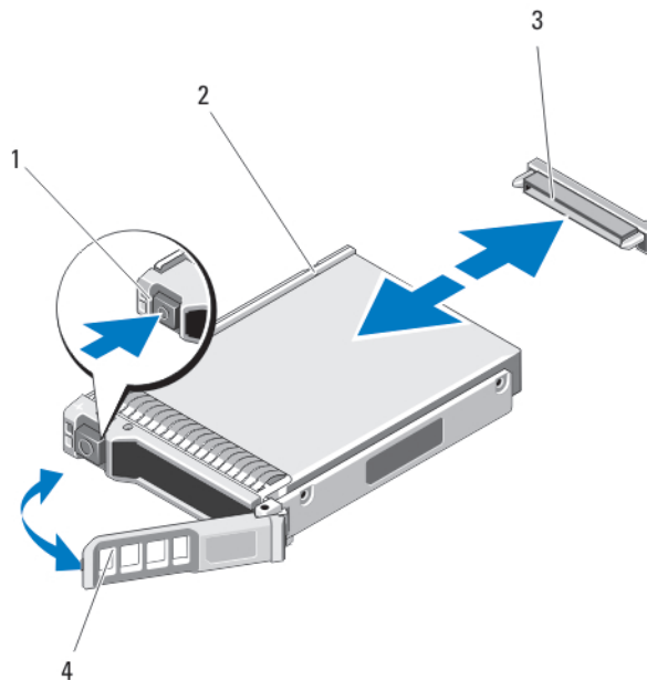
图 19: 卸下和安装硬盘驱动器/SSD
