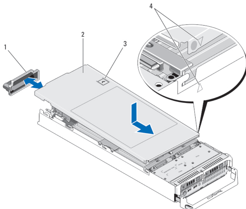
图 6: 打开和合上服务器模块
