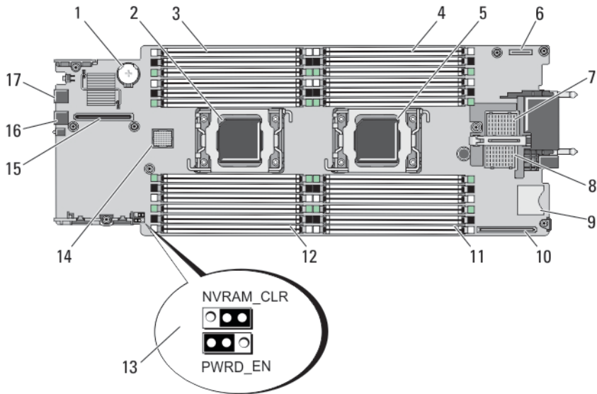
图 25: 系统板连接器
