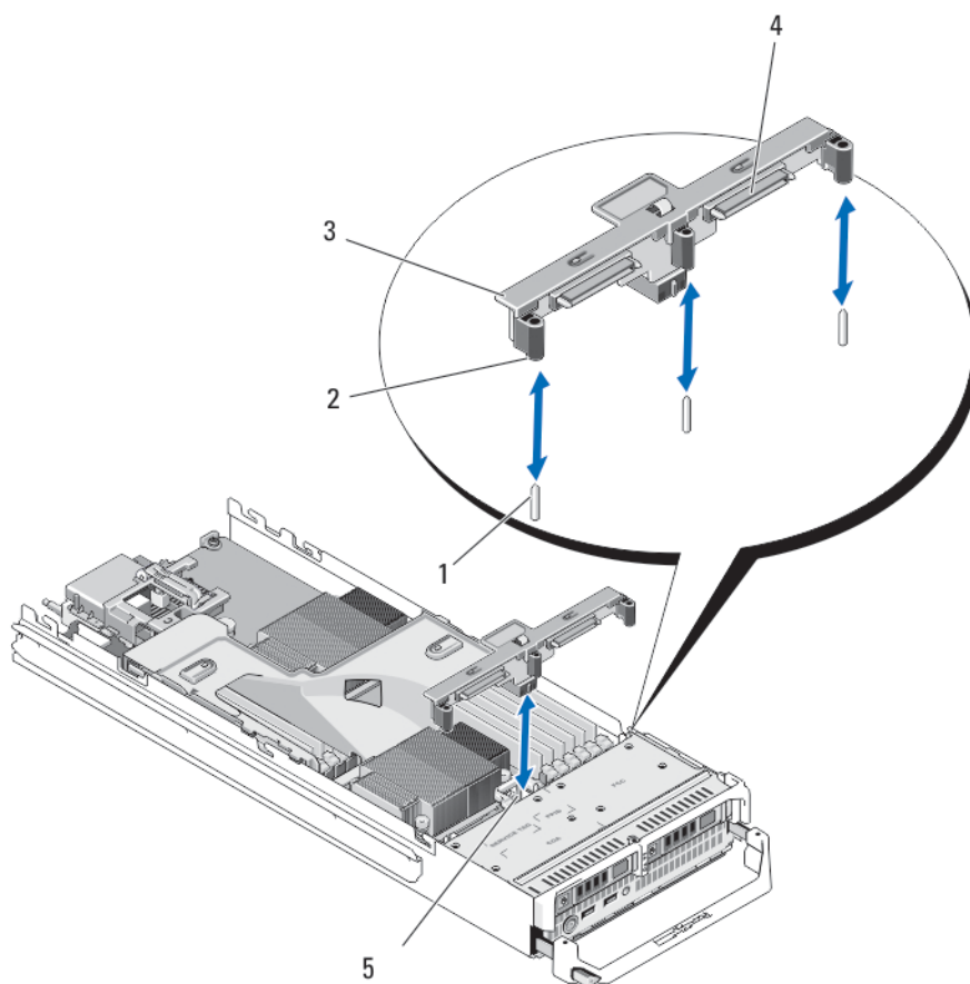
图 21: 卸下和安装硬盘驱动器/SSD 背板
