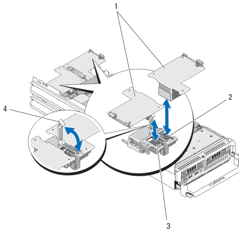
图 11: 卸下和安装 PCIe 夹层卡
