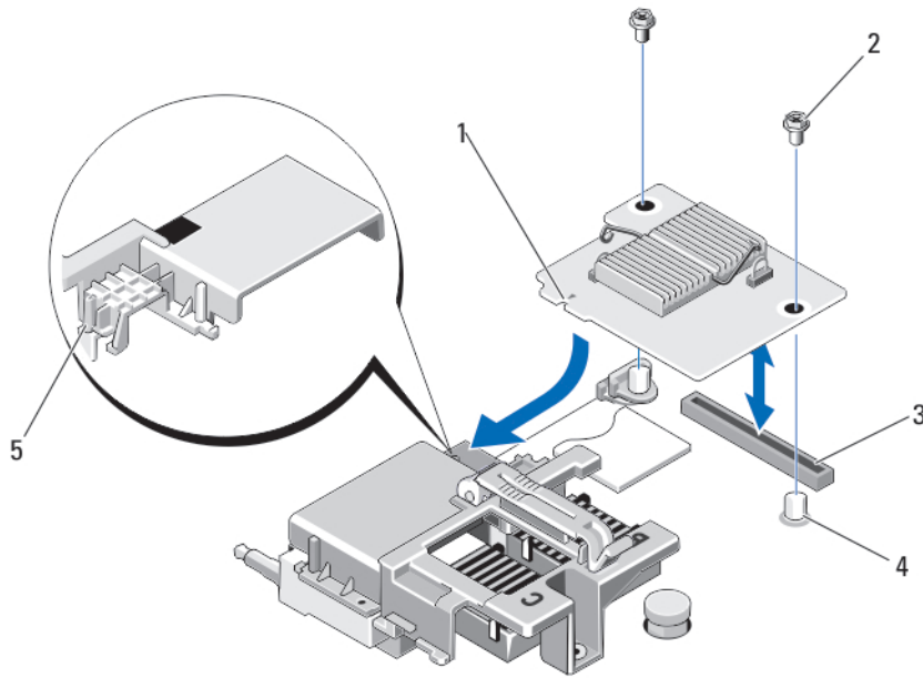
图 15: 卸下和安装网络子卡/LOM 提升卡
