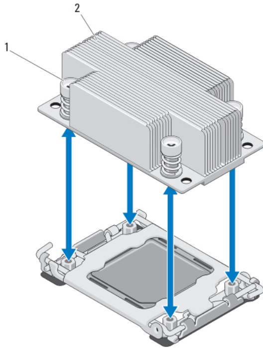
图 16: 安装和卸下散热器
