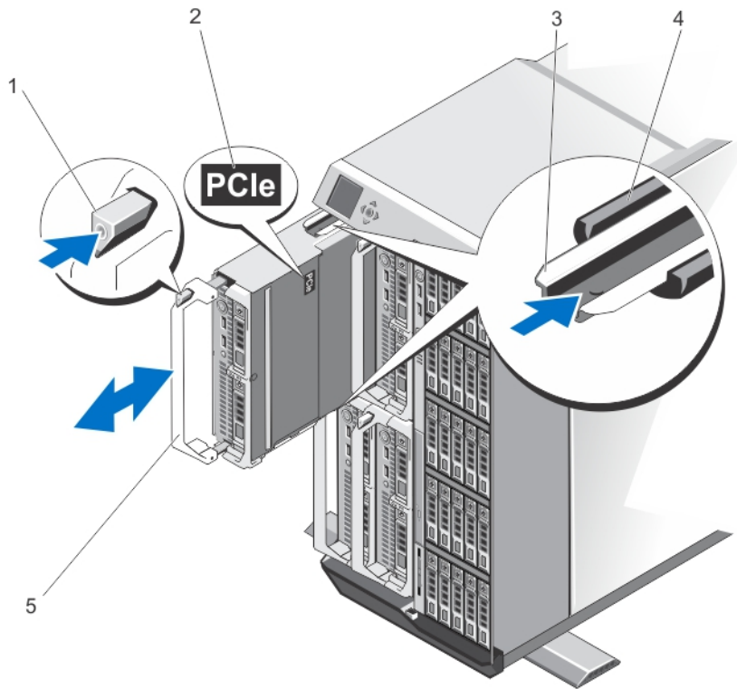
图 5: 卸下和安装服务器模块
