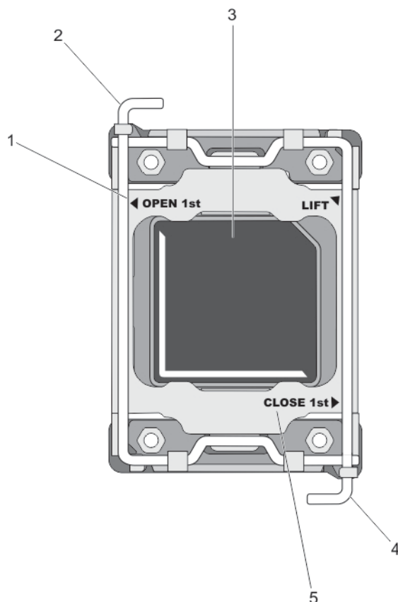
图 17: 处理器护盖打开与合上拉杆的顺序
