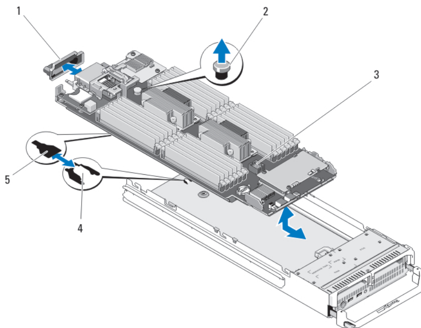
图 22: 卸下和安装系统板
