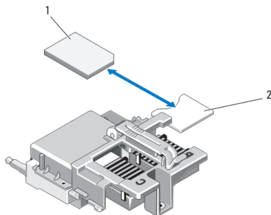
图 14: 装回 SD vFlash 卡
