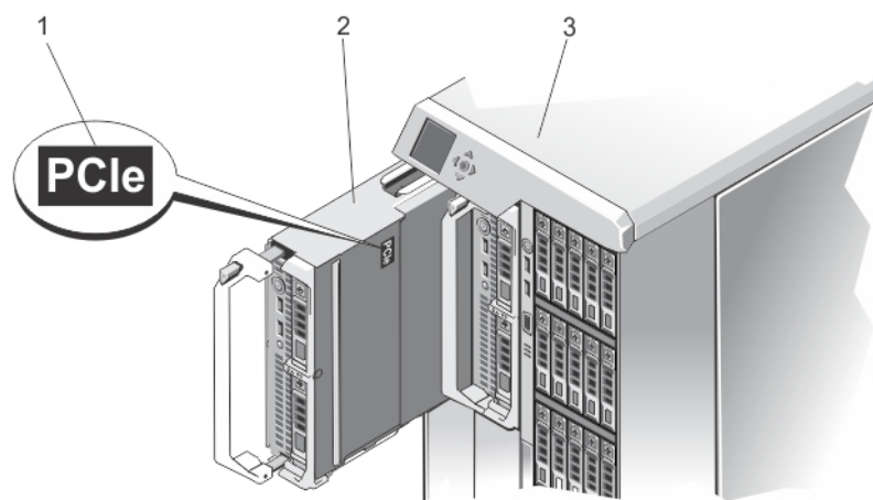
图 1: 识别专为 VRTX 机柜配置的服务器模块
