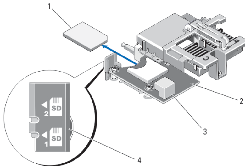
图 12: 更换 SD 卡
