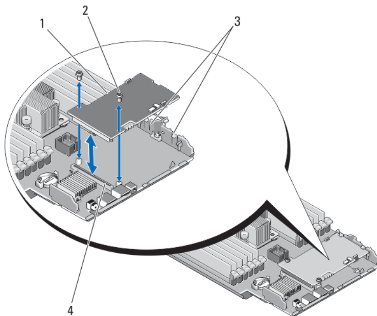
图 24: 卸下和安装存储控制器卡
