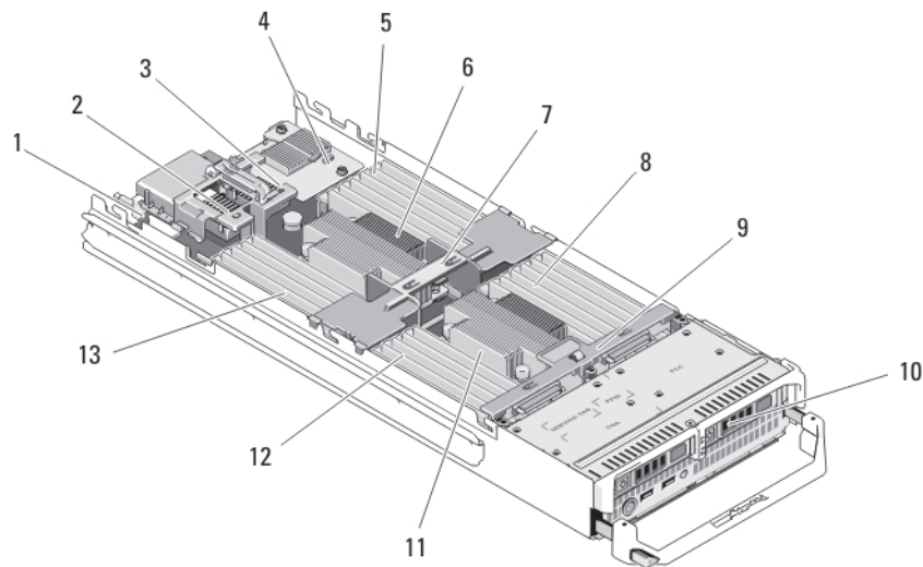
图 7: 服务器模块内部
