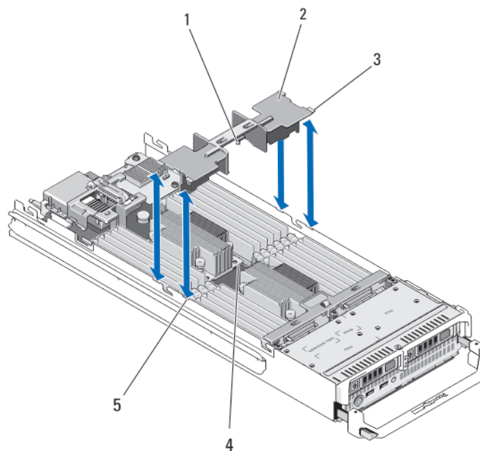
图 8: 安装和卸除冷却导流罩
