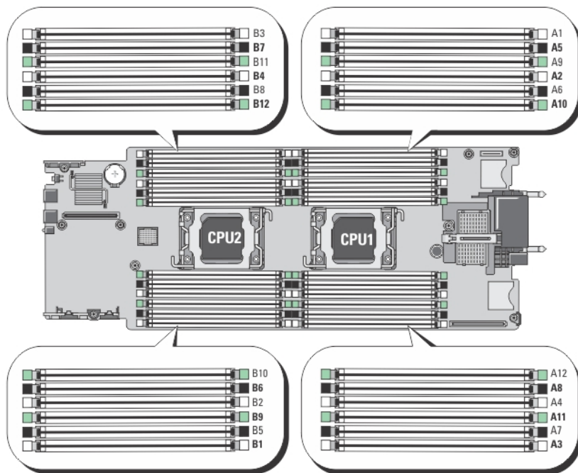
图 9: 内存插槽位置
